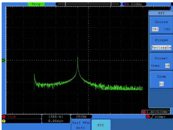
Рисунок 24 - Быстрое преобразование Фурье с прямоугольным окном
