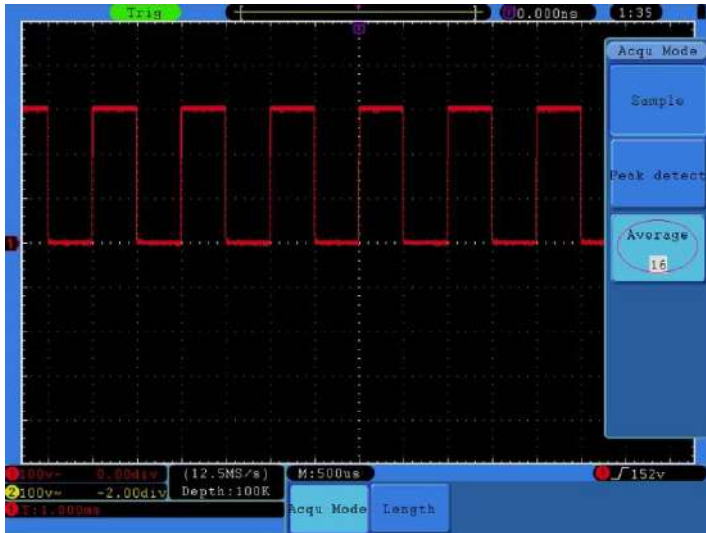
Рисунок 41 - Осциллограмма, на которой шум подавлен в режиме выборки с усреднением по 16 выборкам
