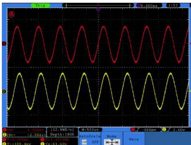
Рисунок 77 - Вид осциллограммы при автоматическом масштабировании по вертикальной и горизонтальной осям с отображением нескольких периодов сигнала
