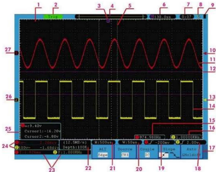
Рисунок 6 - Вид дисплея с интерфейсом пользователя
