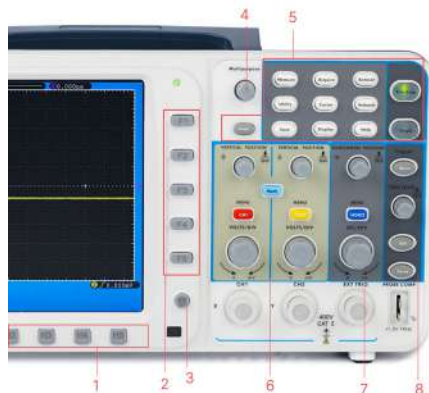
Рисунок 5 - Панель управления
