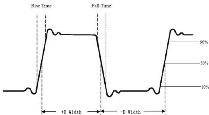
Рисунок 69 - Временные параметры
