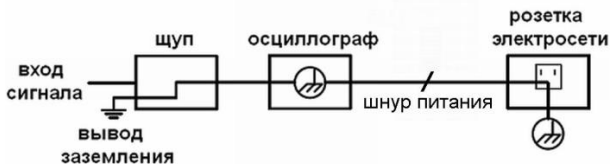
Рисунок 7 - Схема заземления осциллографа
