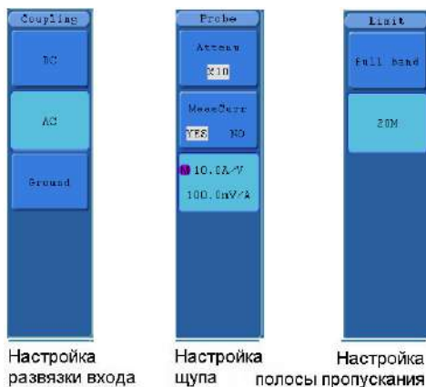
Рисунок 16 - Меню настроек канала
