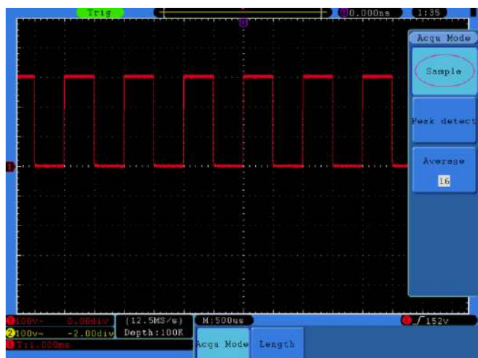
Рисунок 40 - Нормальный режим выборки, при котором помехи на осциллограмме проявляются слабо
