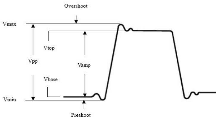
Рисунок 68 - Параметры импульса
