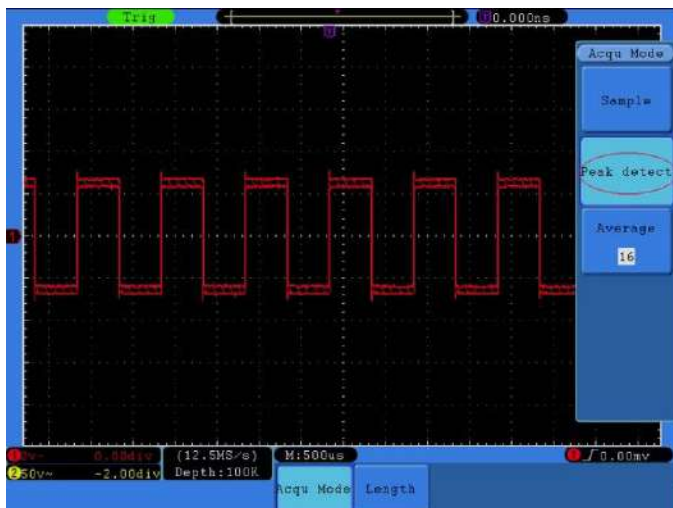
Рисунок 39 - Режим обнаружения пиков, при котором проявляется сильный шум, обнаружены всплески в конце фронтов прямоугольного импульса
