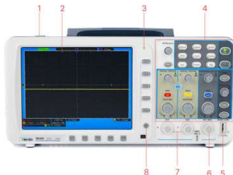
Рисунок 1 - Передняя панель осциллографа
