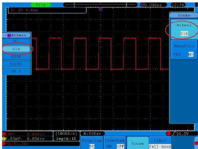
Рисунок 19 - Регулировка коэффициента ослабления щупа
