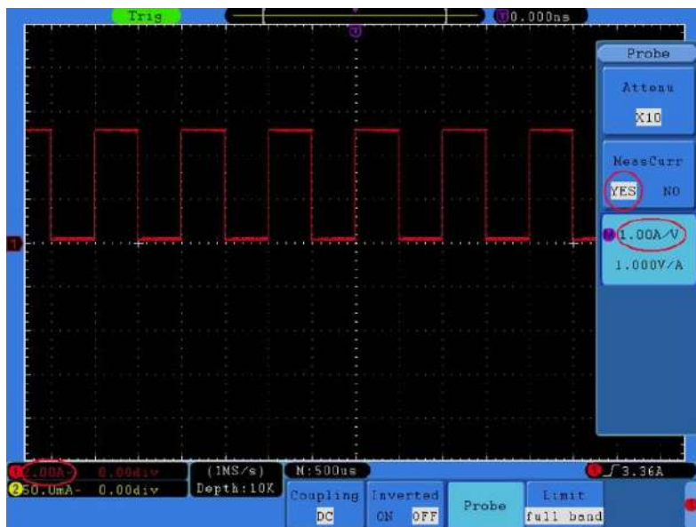
Рисунок 20 - Измерение тока через падение напряжения на резисторе
