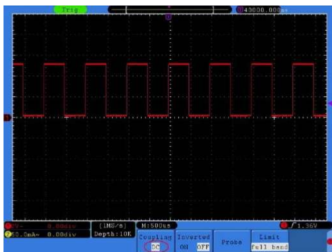
Рисунок 17 - Вид осциллограммы в режиме связи по постоянному току
