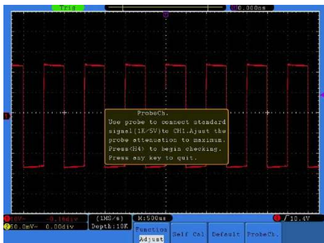
Рисунок 61 - Проверка щупа
