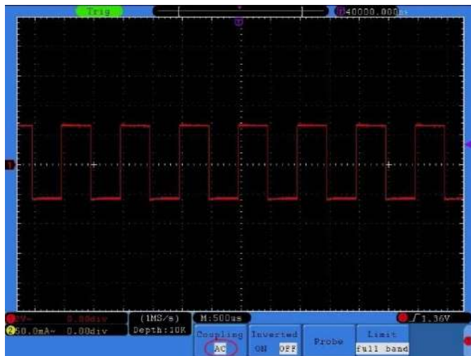
Рисунок 18 - Вид осциллограммы в режиме связи по переменному току
