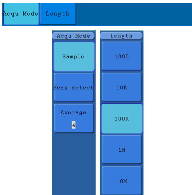
Рисунок 38 - Меню настройки способа выборки ACQU MODE
