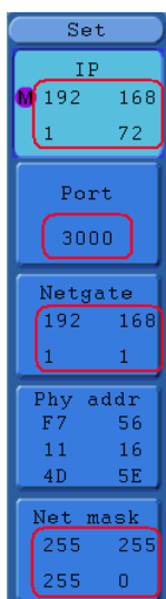
Рисунок 88 - Настройка сетевых параметров осциллографа
