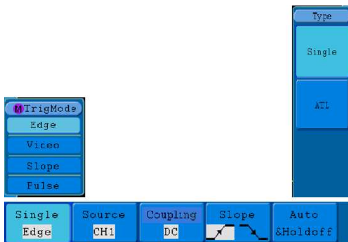
Рисунок 30 - Меню запуска по фронту
