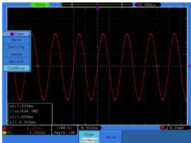
Рисунок 50 - Вырезание осциллограммы
