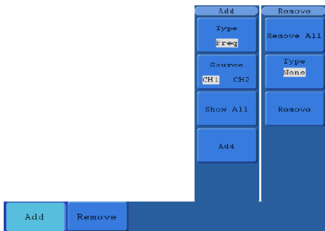
Рисунок 66 - Меню настройки автоматических измерений
